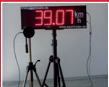
Schusskraft Messung
